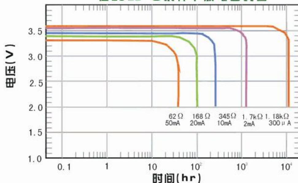
在不同电流,温度条件下容量曲线图
