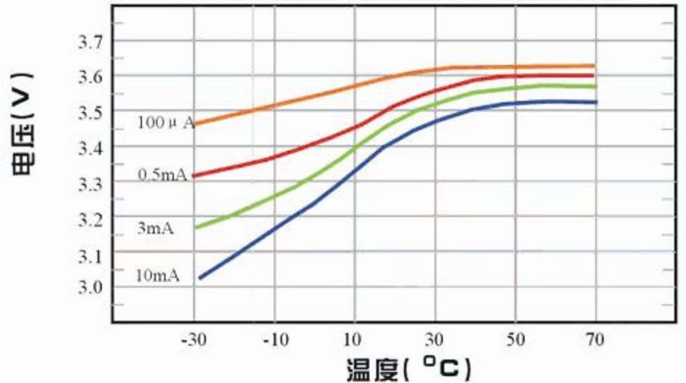
在不同温度,电流条件下电压曲线图
